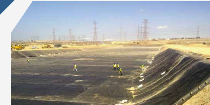
BASSIN PROVISoire DE FLOTTAISON CONDUITES OCP JORF LASFAR
